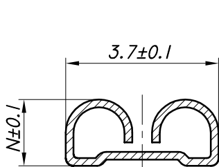
CORTE V-V
