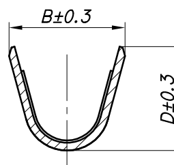
CORTE U-U
