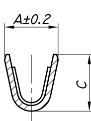
CORTE P-P
